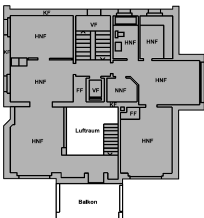
Grundriss 1. Obergeschoss:
