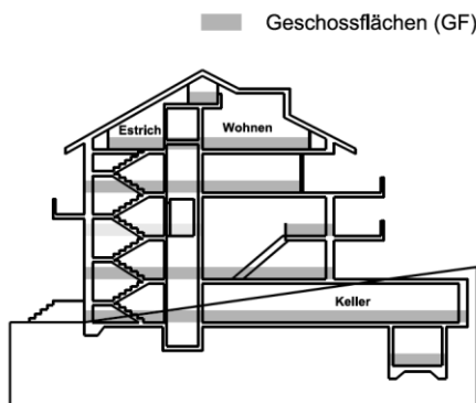
Schnitt:
